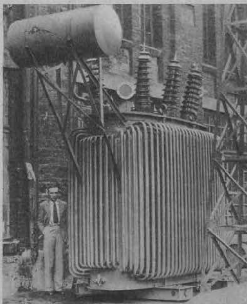
Największy w Polsce transformator, wykonany w łódzkich warsztatach sp. akc. „Elektrobudowa”, o mocy 3000 KVA na napięciu: 60000 \pm 5/15.000/16.250/6400 volt, który stanąć ma w Pomorskiej Elektrowni Krajowej Gródek.
