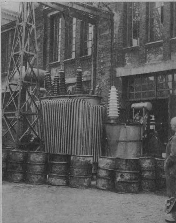
Największy w Polsce transformator, wykonany w łódzkich warsztatach sp. akc. „Elektrobudowa”, o mocy 3000 KVA na napięciu: 60000 \pm 5/15.000/16.250/6400 volt, który stanąć ma w Pomorskiej Elektrowni Krajowej Gródek.
