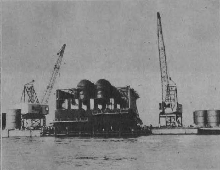
Olbrzymia konstrukcja przy budowie mostu w San Francisco, pozwalająca na pracę 30 m. pod poziom wody.
