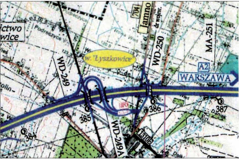
Projekt węzła autostradowego w Łyszkowicach.
