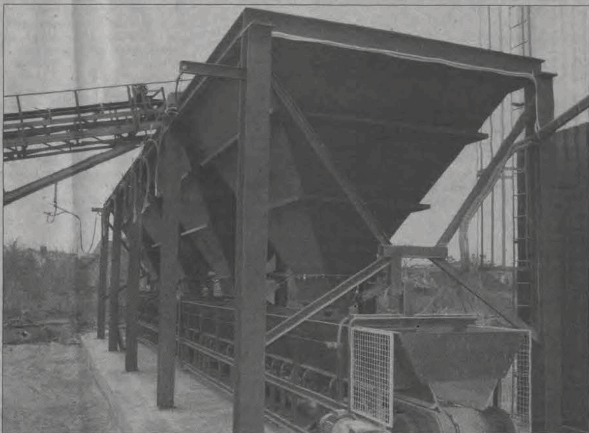
Wraz z nową linią zamontowany został też nowy węzeł betoniar-ski.
